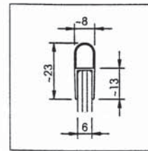
Art. 230.000 Streifendichtung für 6 mm Glas Nr. 1006520
