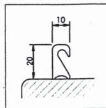
Art. 205.000 Plexi Wellenbrecher, gerade
