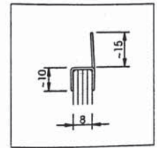
Art. 254.000 H-Profil mit weicher Lippe, groß, für 8 mm Glas Nr. 1002739
