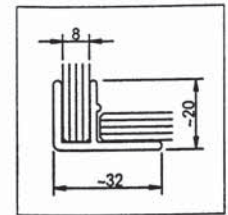
Art. 207.000 Abdichtprofil für 8 mm Glas Nr. 1002743
