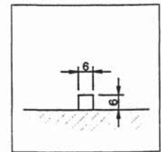
Art. 200.000 Plexi vierkant 6 x 6 mm
