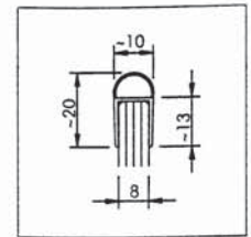
Art. 226.000 Streifendichtung für 8 mm Glas Nr. 1003384
