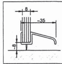
Art. 250.000 Tür Abtropfprofil für 8 mm Glas Nr. 1002738
